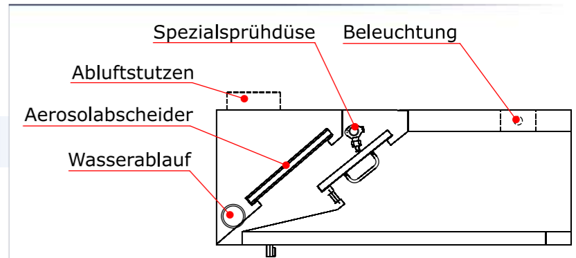
Schnitt durch eine selbstreinigende Ablufthaube
